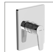
HANSAPOLO súprava na hotovú montáž s funkčnou jednotkou páková sprchová batéria HANSABLUEBOX funkčná jednotka s dekoráčnou súpravou (1) 8061 9093 chróm bezskrutková ružica, funkčná jednotka bez prepínania
